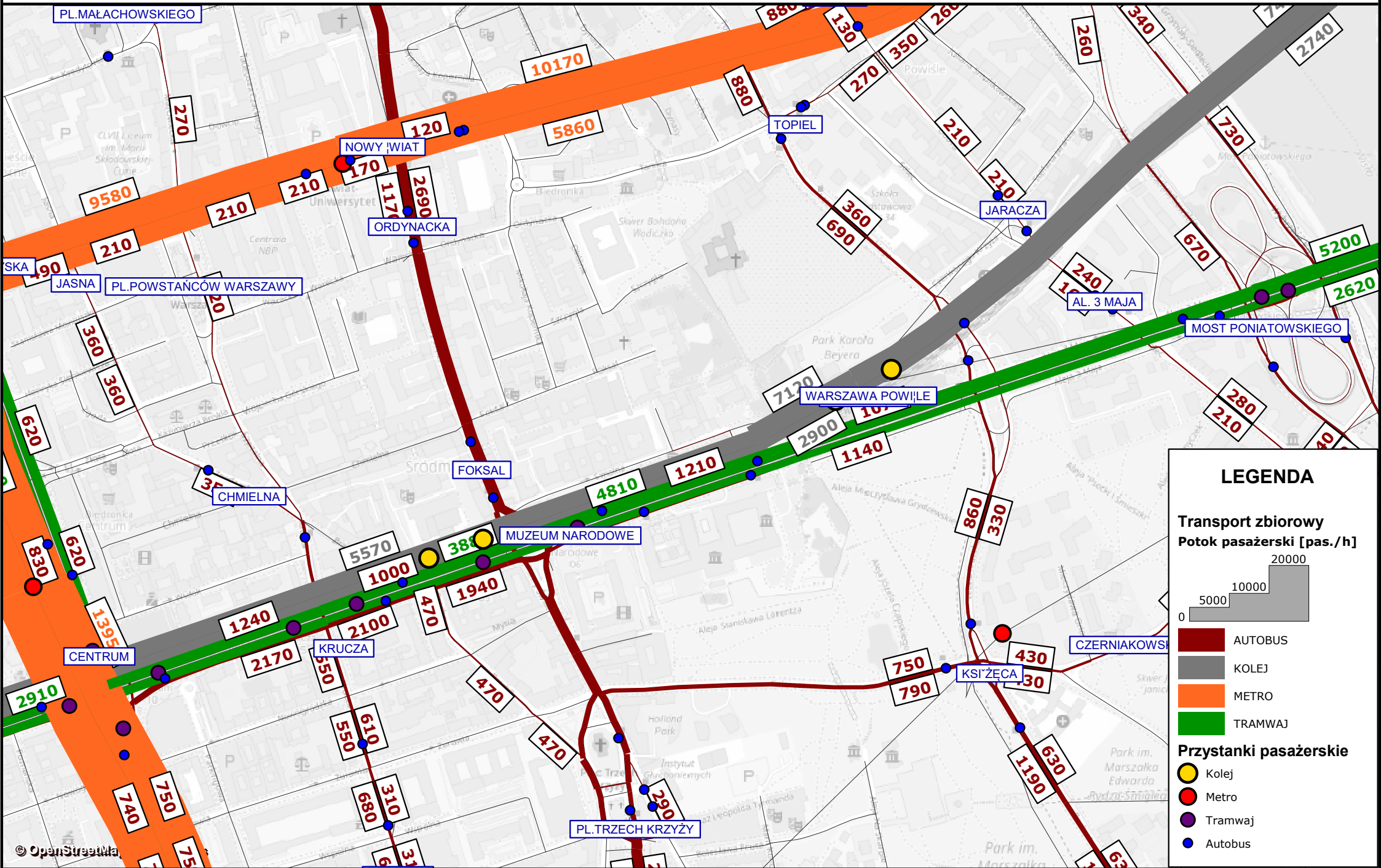
POTOKI PASAŻERSKIE W SZCZYTY PORANNYM - 11 2025
