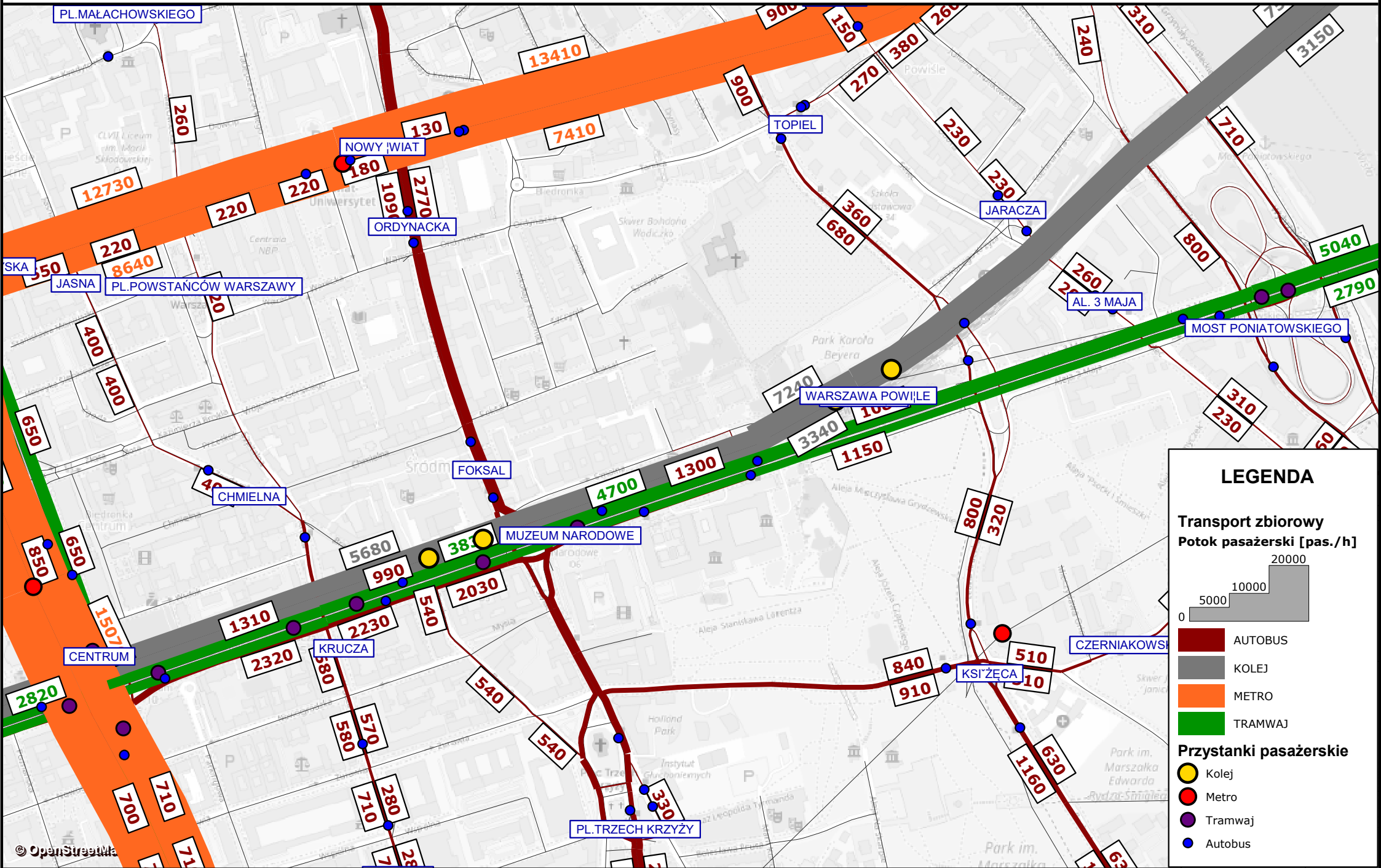
POTOKI PASAŻERSKIE W SZCZYCIE PORANNYM - 11 2035
