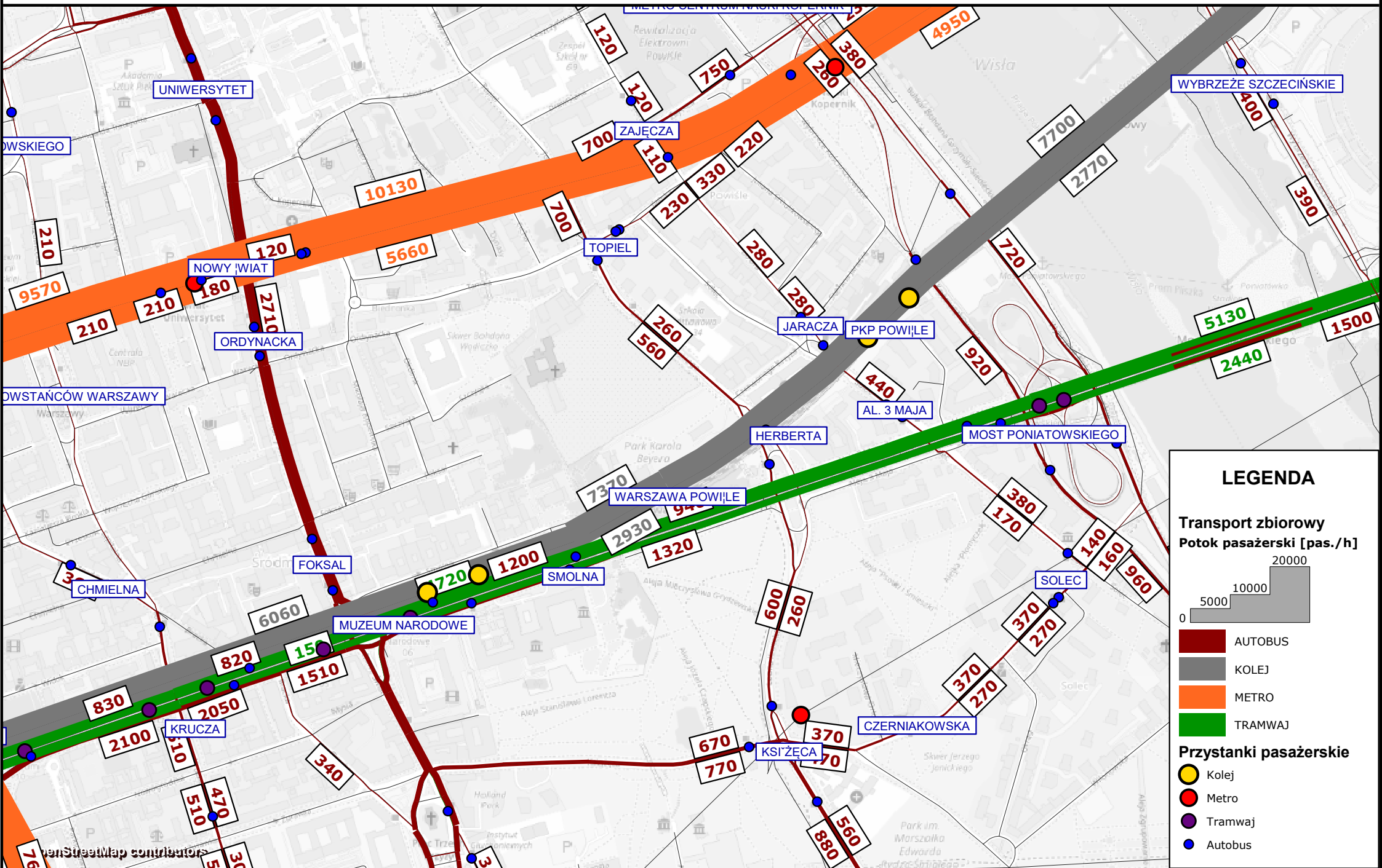
POTOKI PASAŻERSKIE W SZCZYTCIE PORANNYM - I2a 2025
