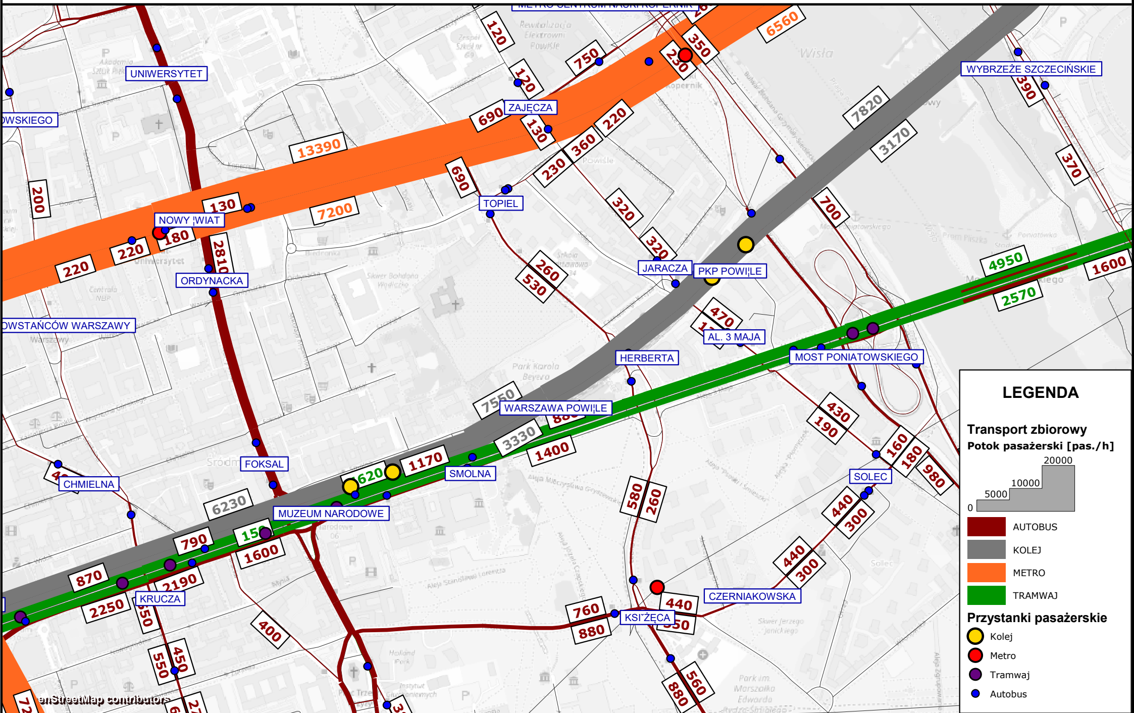
POTOKI PASAŻERSKIE W SZCZYTCIE PORANNYM - I2a 2035
