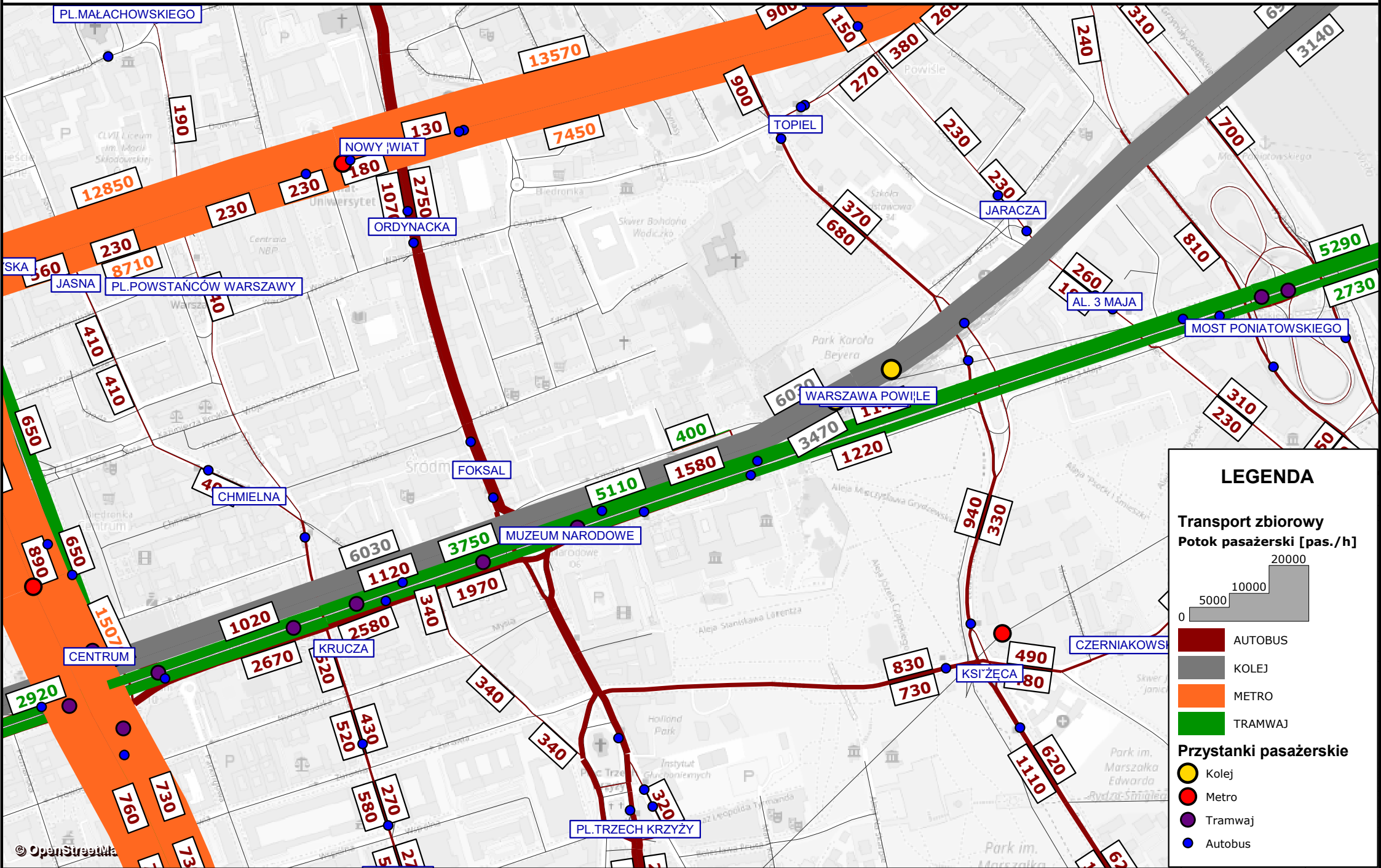
POTOKI PASAŻERSKIE W SZCZECIE PORANNYM - 10 2035
