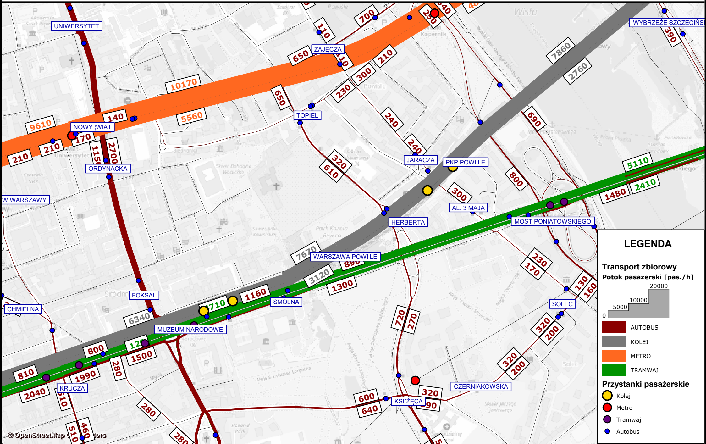
POTOKI PASAŻERSKIE W SZCZYTCIE PORANNYM - 12b 2025
