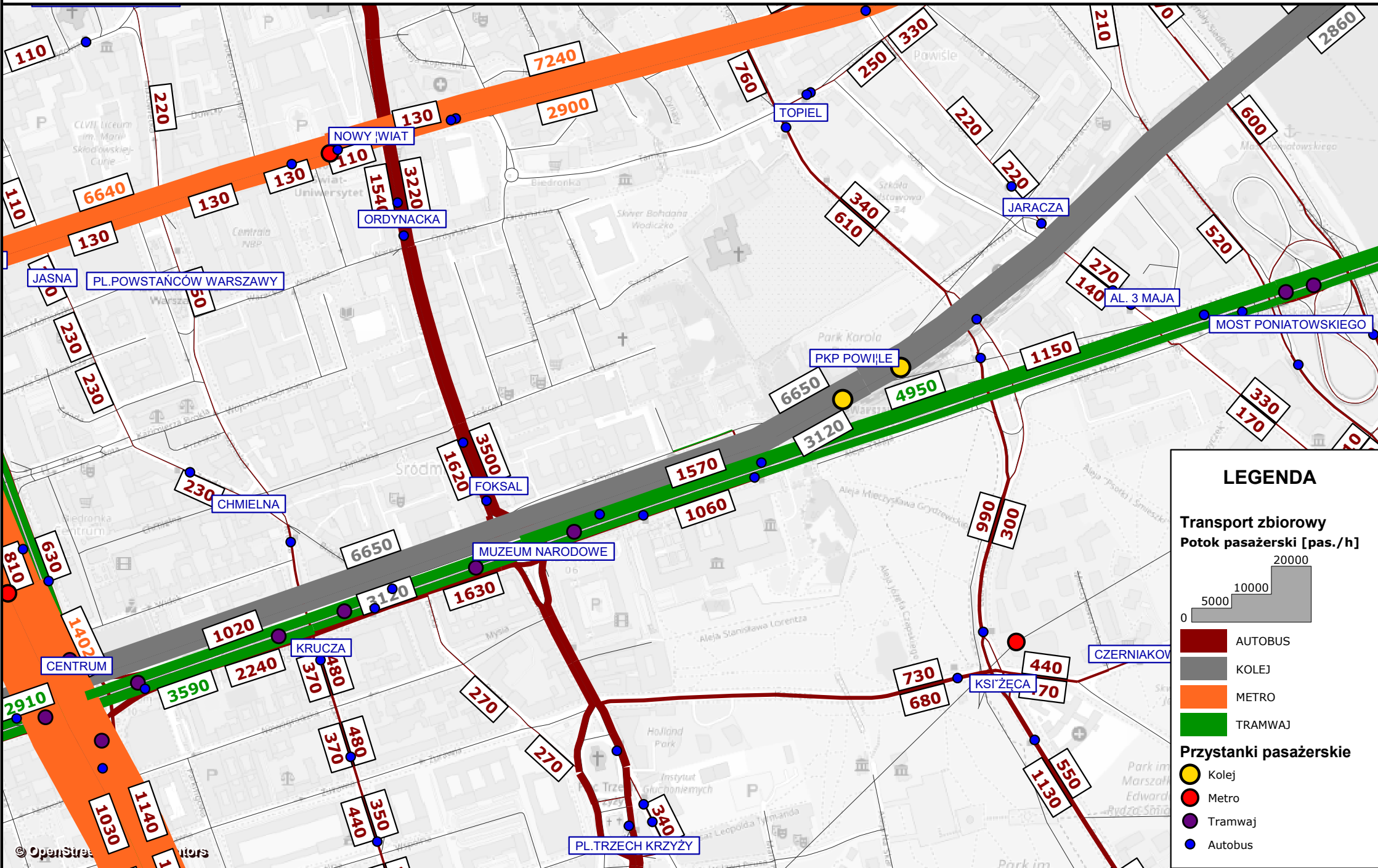
POTOKI PASAŻERSKIE W SZCZYTY PORANNYM - 10 2016
