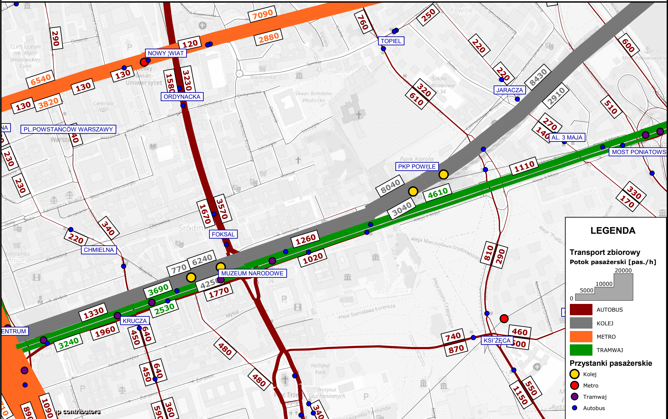
POTOKI PASAŻERSKIE W SZCZYCIE PORANNYM - 11 2016
