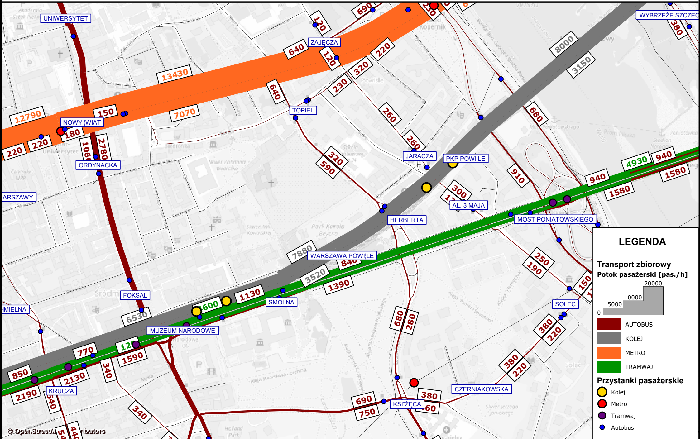
POTOKI PASAŻERSKIE W SZCZYPIE PORANNYM - 12b 2035
