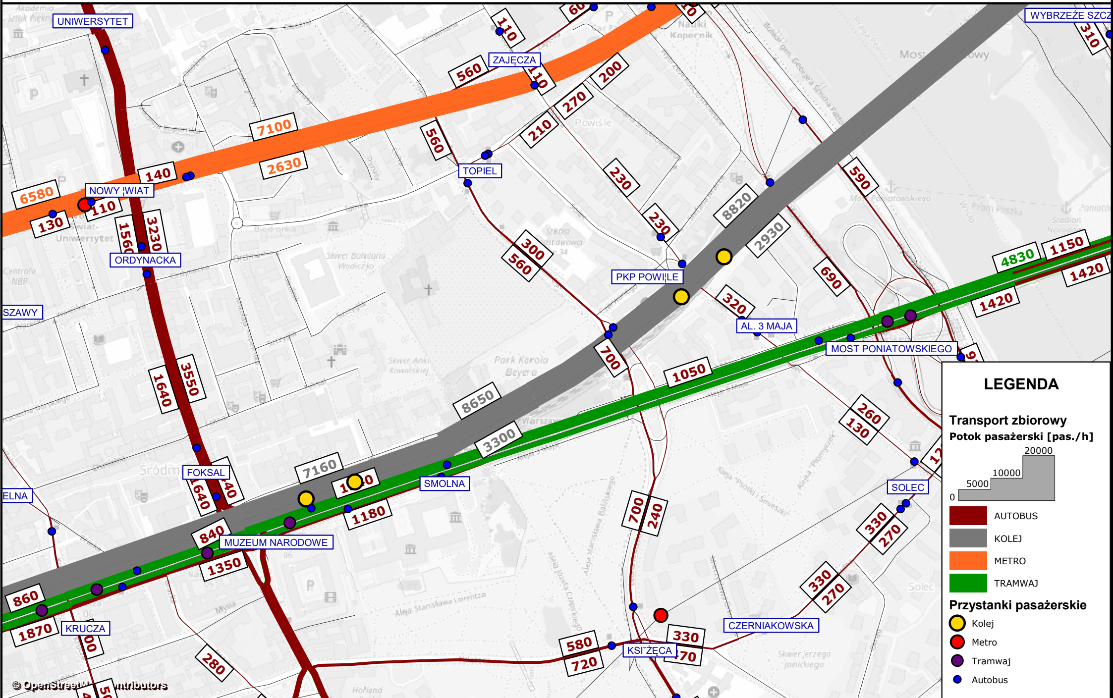
POTOKI PASAŻERSKIE W SZCZYTY PORANNYM - 12b 2016
