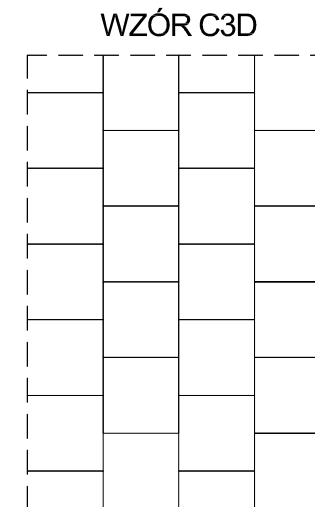
PŁYTY BETONOWE SZARE O WYMIARACH: 50 x 50 cm UKŁADANE PASAMI Z PRZESUNIĘCIEM 1/2
