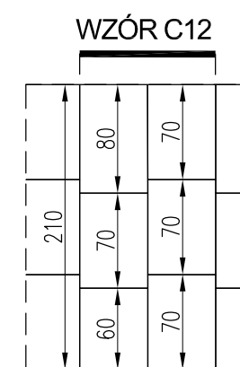
PLYTY BETONOWE O WYM. 60, 70, 80 x 50 cm
