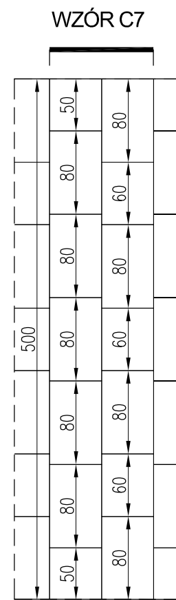
PŁYTY BETONOWE SZARE O WYM. 50, 60, 80 x 50 cm
