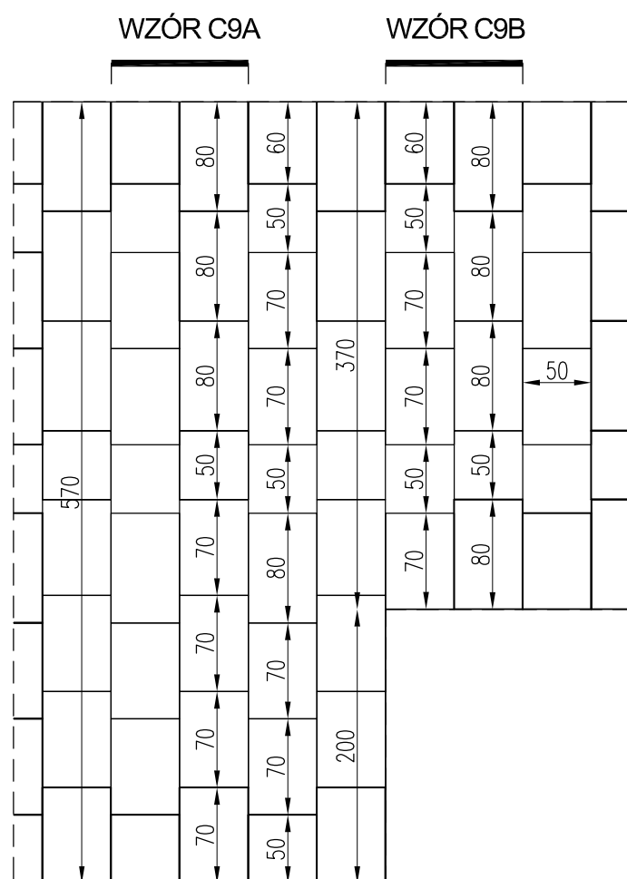
PLYTY BETONOWE SZARE O WYM. 50, 60, 70, 80 x 50 cm
