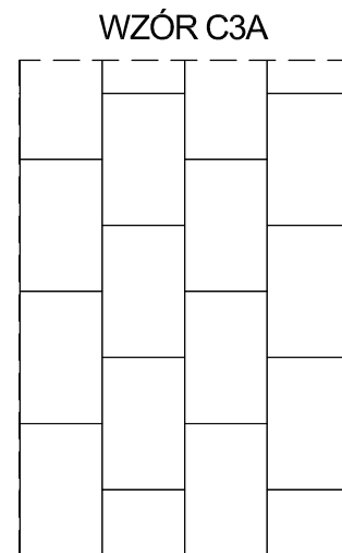
PŁYTY BETONOWE SZARE O WYMIARACH: DŁUGOŚĆ 80 cm SZEROKOŚĆ 50 cm UKŁADANE PASAMI Z PRZESUNIĘCIEM 1/2
