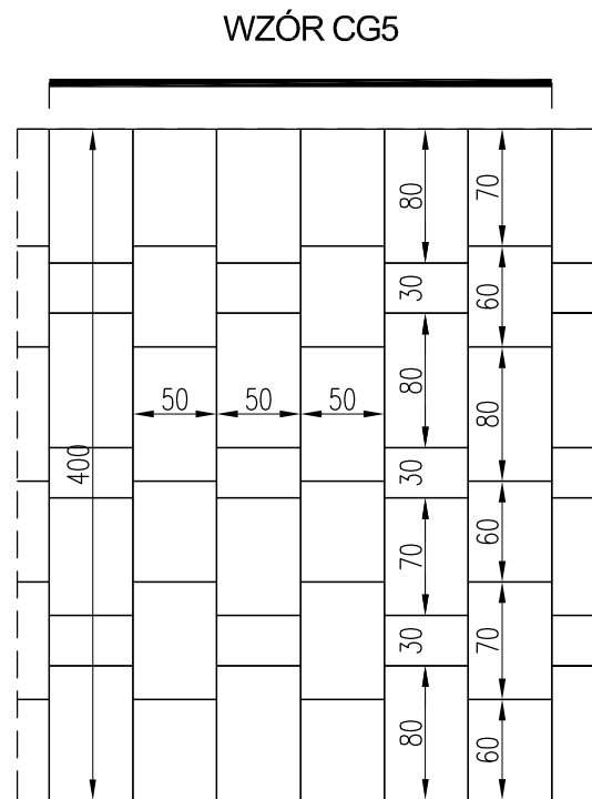
PŁYTY GRANITOWE GROSZKOWANE SZARE O WYM. 30, 60, 70, 80 x 50 cm
