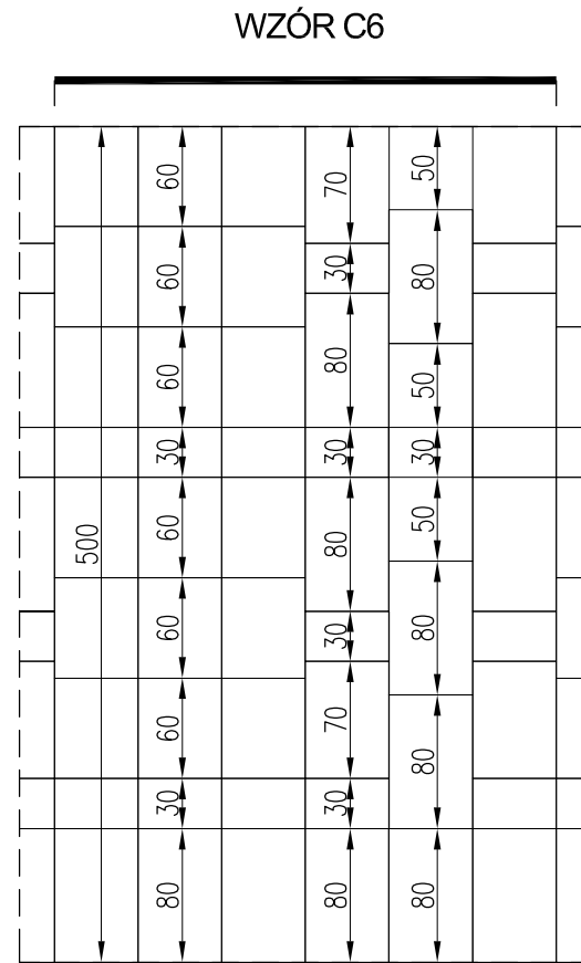
PŁYTY BETONOWE SZARE O WYM. 30, 60, 70, 80 x 50 cm
