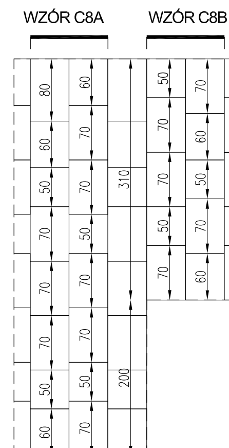
PŁYTY BETONOWE SZARE O WYM. 50, 60, 70, 80 x 50 cm
