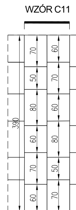
PLYTY BETONOWE O WYM. 50, 60, 70, 80 x 50 cm
