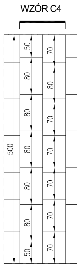
PŁYTY BETONOWE SZARE O WYM. 50, 60, 70, 80 x 50 cm
