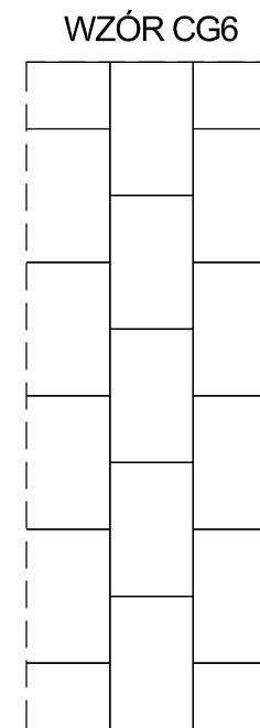
PŁYTY GRANITOWE GROSZKOWANE SZARE O WYMIARACH: DŁUGOŚĆ 80 cm SZEROKOŚĆ 50 cm UKŁADANE PASAMI Z PRZESUNIĘCIEM 1/2
