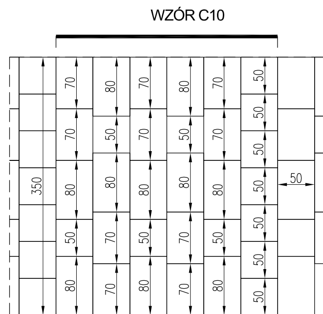
PLYTY BETONOWE O WYM. 50, 70, 80 x 50 cm
