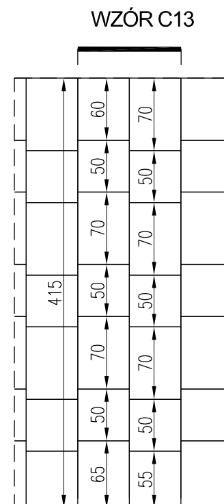
PLYTY BETONOWE O WYM. 50, 55, 60, 65, 70 x 50 cm
