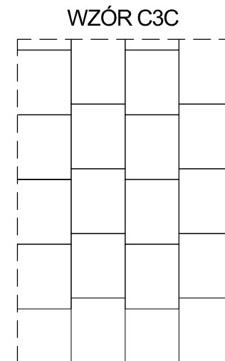
PŁYTY BETONOWE SZARE O WYMIARACH: DŁUGOŚĆ 60 cm SZEROKOŚĆ 50 cm UKŁADANE PASAMI Z PRZESUNIĘCIEM 10/50 cm
