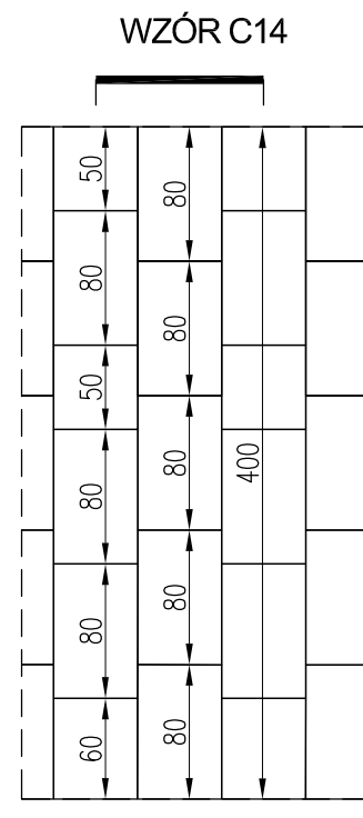
PLYTY BETONOWE SZARE O WYM. 50, 60, 80 x 50 cm
