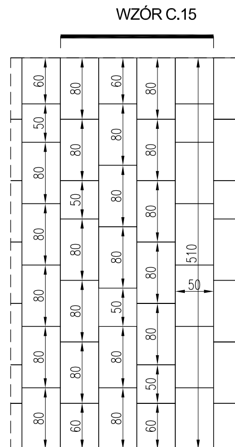
PLYTY BETONOWE SZARE O WYM. 50, 60, 80 x 50 cm
