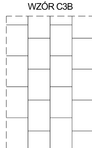
PŁYTY BETONOWE SZARE O WYMIARACH: DŁUGOŚĆ 70 cm SZEROKOŚĆ 50 cm UKŁADANE PASAMI Z PRZESUNIĘCIEM 1/2
