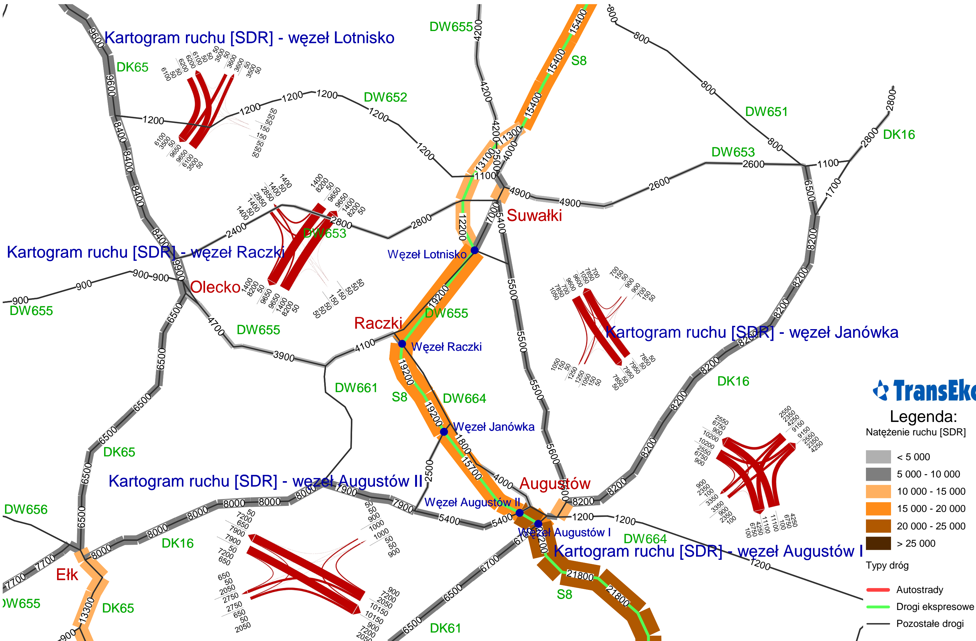
Kartogramy ruchu na węzłach obwodnicy Augustowa w Wariancie III (Raczki) - Rok 2020. Rys. 6.5
